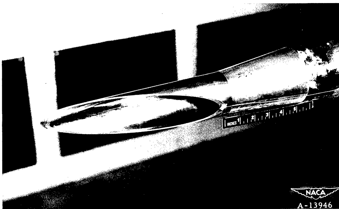
(d) 75°-bevelled outlet.
