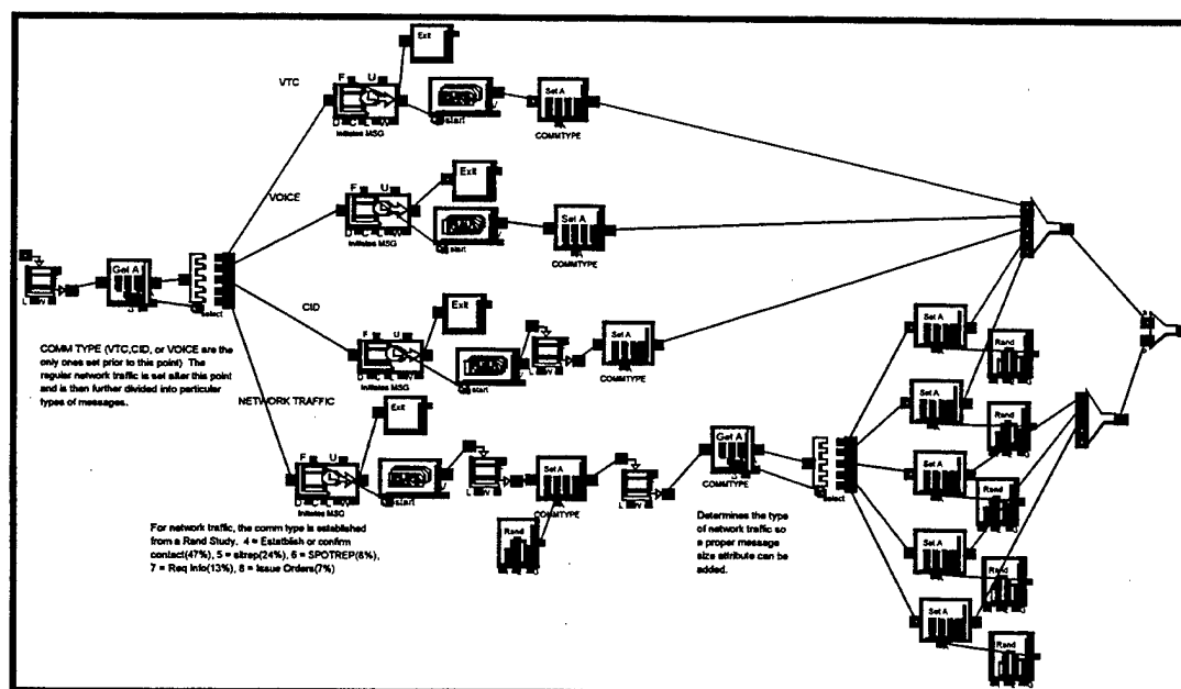
Figure 11. MSG Routing
