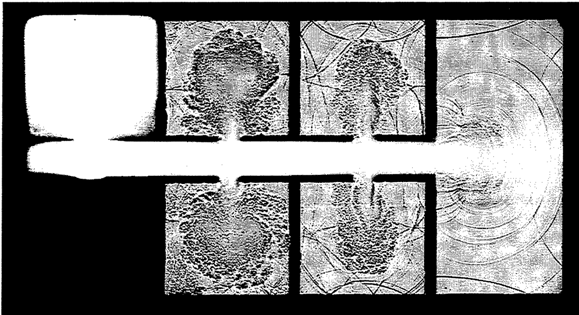
b) W = 0.52 \text{ g NP} + 0.06 \text{ g Al} (test 15432)
