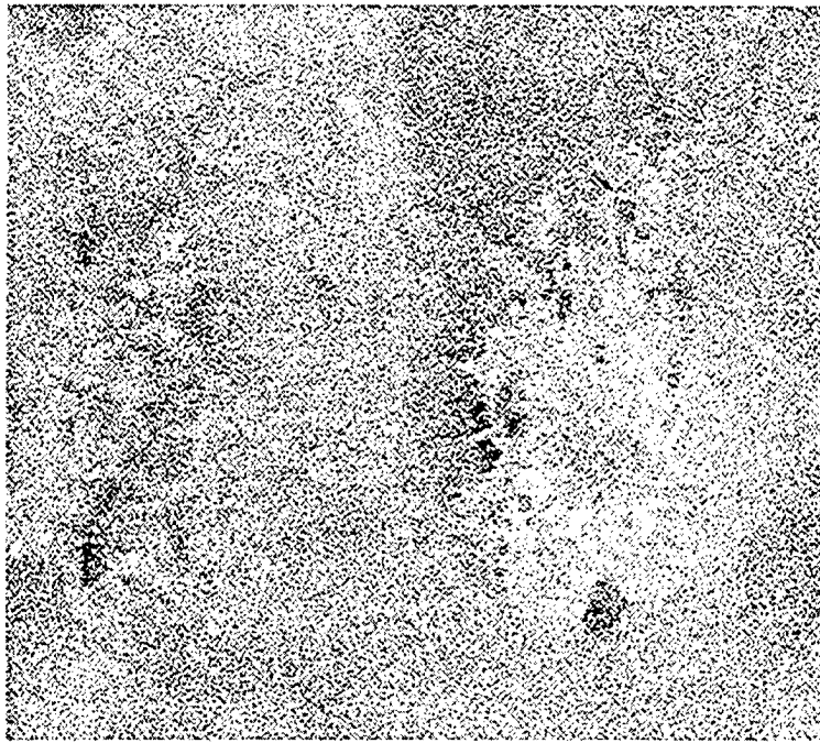
Fig. 4.4 (d) Band Nine of sample PC Rotation
