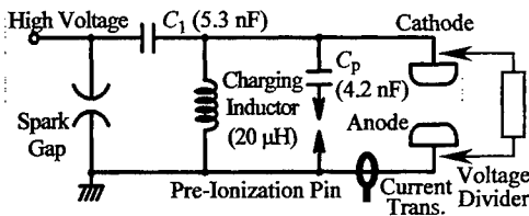
(d) Electrical excitation circuits.
