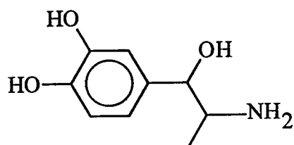
Levonordefrine
