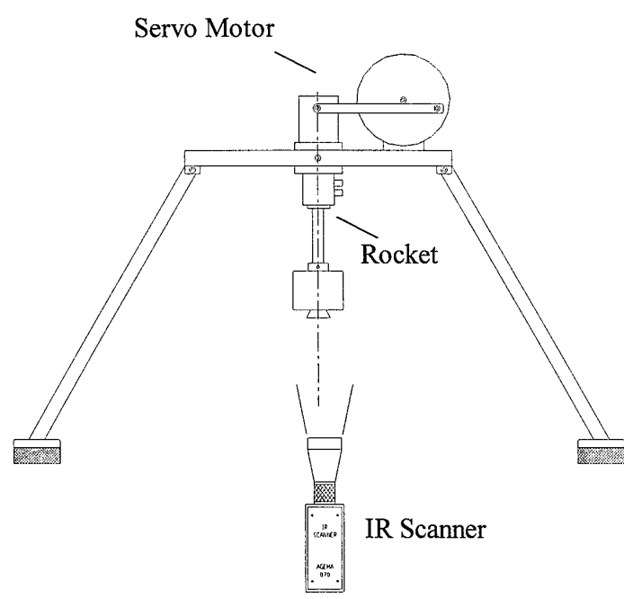
Fig. 1. Spinning rocket test stand
