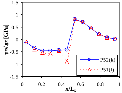
(d) Shear stress ( t_{xz} ) with a_2 = 0
