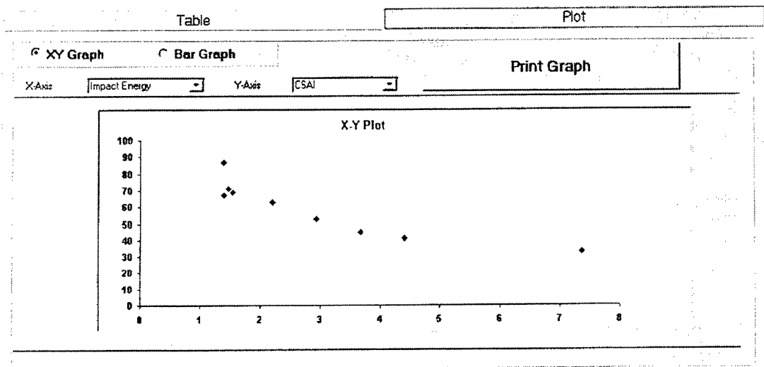
FIGURE 25. IMPACT ENERGY (ft-lb) VERSUS CSAI (ksi) GRAPH UNDER THE SPECIFIED PARAMETERS OF CASE 6.1.1
