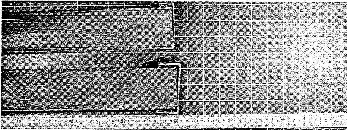
Figure D.27. Core H, 128-160 cm.
