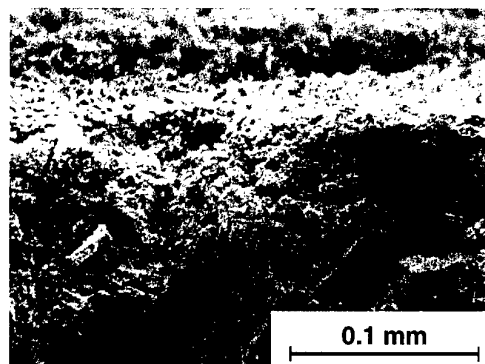
SEM fractograph (Wanhill et al. 1995)
