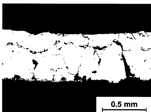
Intergranular: metallograph (Werner 1965)
