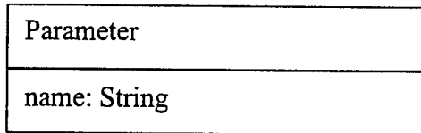
Figure 27 – Parameter Type
