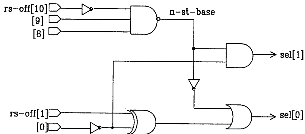
super-ctrl/read-mux-ctrl
