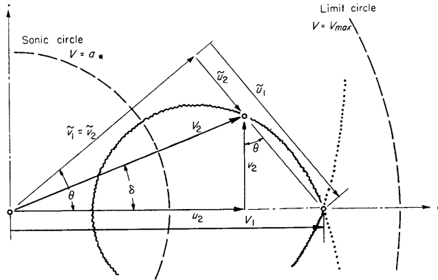
FIGURE 3.—Shock polar.
