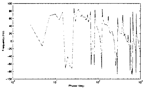
G_{y2u2} : PZT2-to-Mic2
