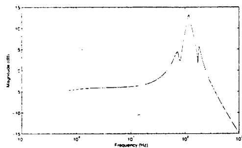
G_{u_1y_1} : Mic1-to-PZT1
