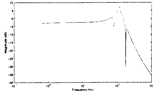
G_{u_1y_2} : Mic2-to-PZT1
