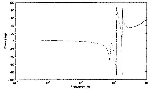
G_{u_2y_2} : Mic2-to-PZT2
