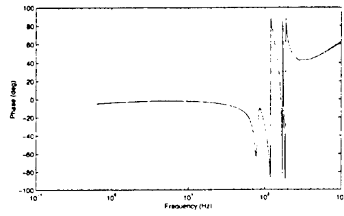
G_{u_1y_2} : Mic2-to-PZT1
