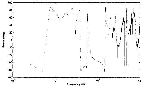
G_{yw} : Mic2-to-Mic1
