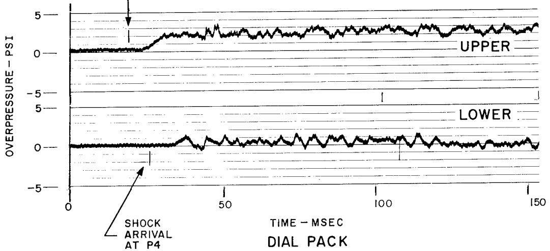
Figure 3.12. --Plenum overpressures.
