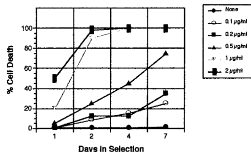
B. Zeocin cytotoxicity
