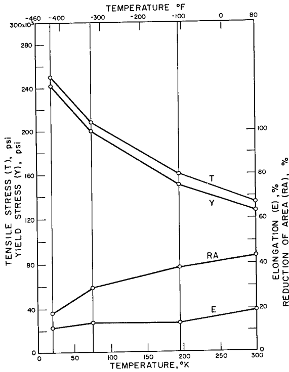
Ti 5Al - 2.5 Sn, ANNEALED
