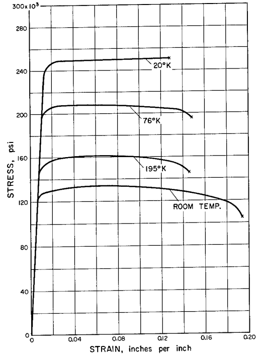
Ti 5Al - 2.5 Sn, ANNEALED
