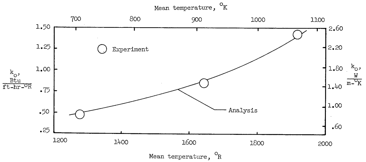
(d) \lambda = 5 .
