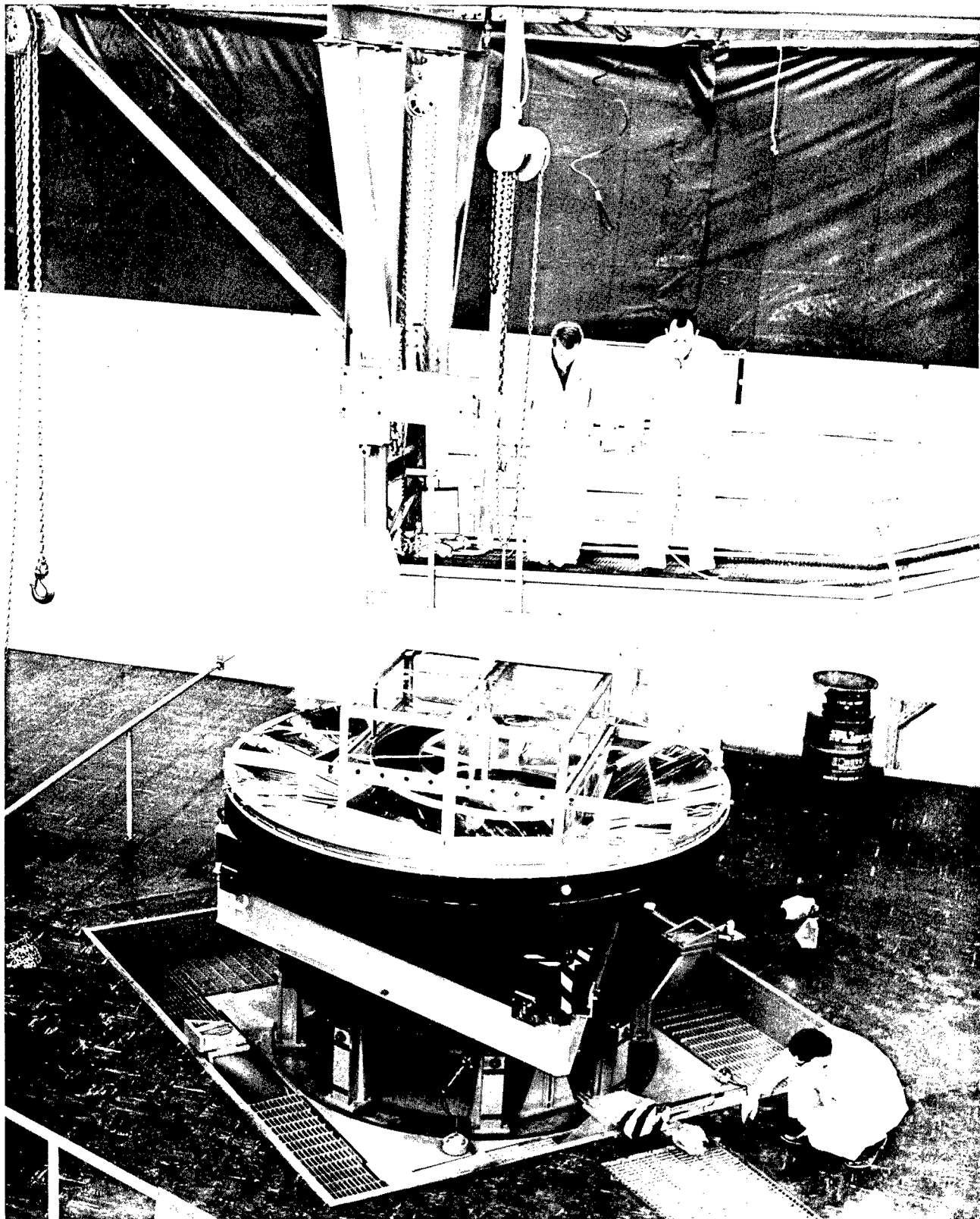
Figure 5.2-7. Spincasting of Pour No. 3
