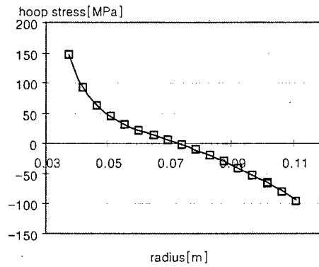
(d) hoop stress of cylinder B
