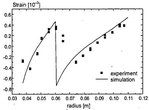
(d) hoop strain of Specimen B
