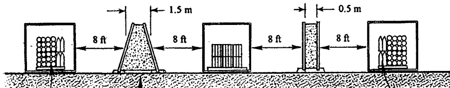
ELEVATION
