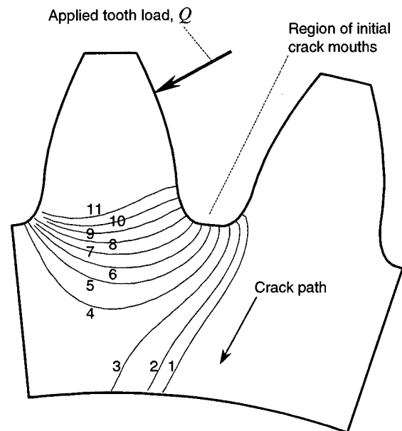
Fig. 5. Effect of initial crack location on crack propagation path, m_b=1.0 , 1) \theta_o=68^\circ , 2) \theta_o=73^\circ , 3) \theta_o=78^\circ , 4) \theta_o=83^\circ , 5) \theta_o=88^\circ , 6) \theta_o=94^\circ , 7) \theta_o=99^\circ , 8) \theta_o=104^\circ , 9) \theta_o=109^\circ , 10) \theta_o=114^\circ , 11) \theta_o=120^\circ .
