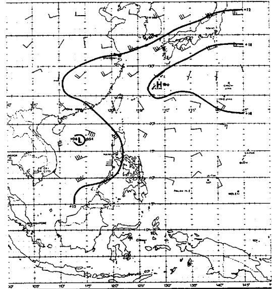
b. 700mb ANAL
