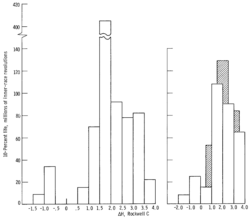
(b) Actual \Delta H increment, 1.0.
