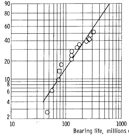
(d) Ball Rockwell C hardness, 66.
