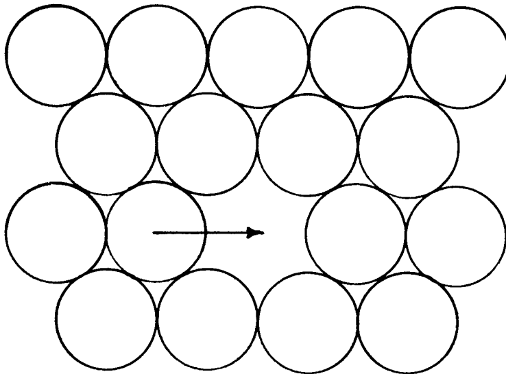
Figure 1-2. Vacancy Diffusion
