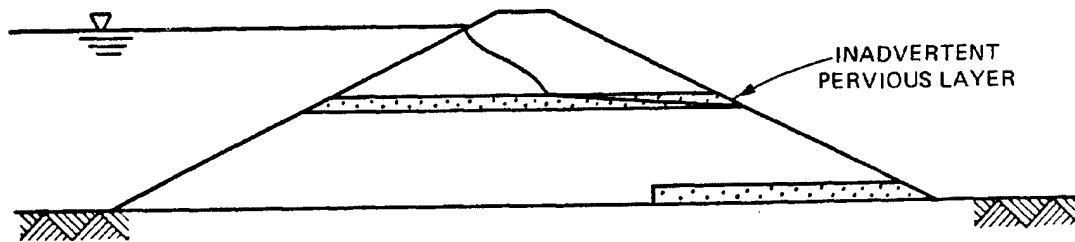
a. HORIZONTAL DRAIN ONLY
