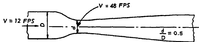
a. VENTURI METER
