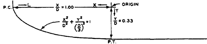
a. SIMPLE CURVES
