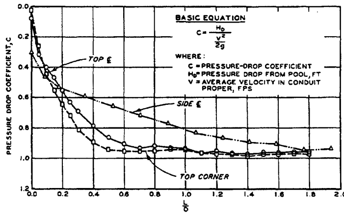
a. SIMPLE CURVES
