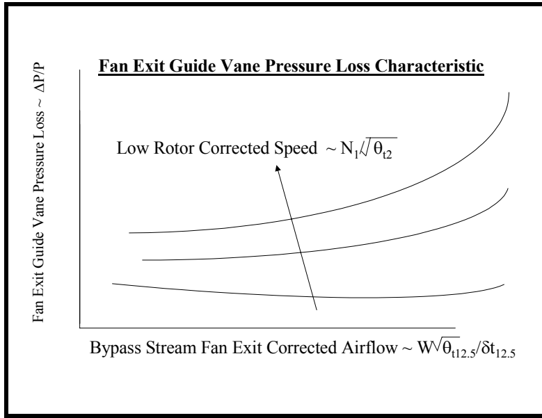
Figure 32 - Fan exit guide vane (FEGV) map
