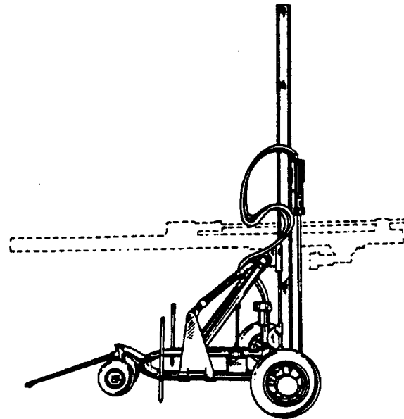
Fig. 4-11. Wagon drill 9
