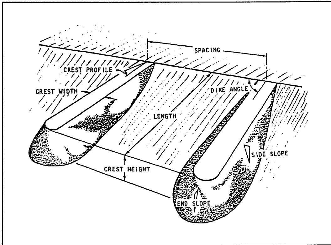
Figure 7-3. Stone spur dike parameters
