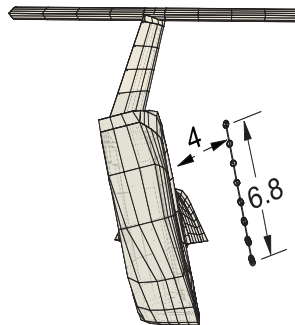
(d) Rear view of fan measurement locations.
