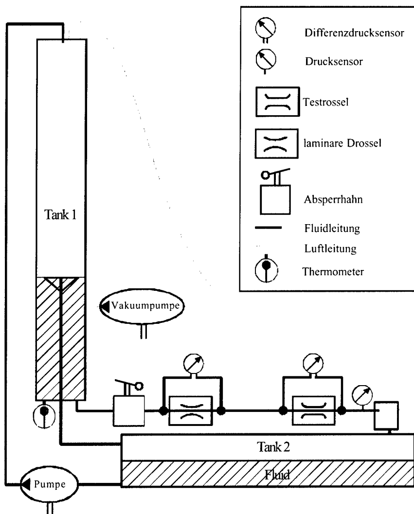
Abbildung 7.1: Skizze der Messapparatur.
