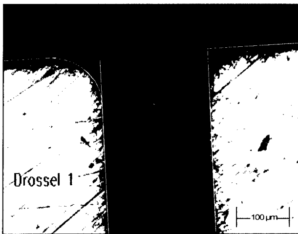
Abbildung 6.13: Profil der Einlasskante einer Drossel im Maßstab 200:1. Der Radius der Verrundung beträgt ca. 100 \mu\text{m} .
