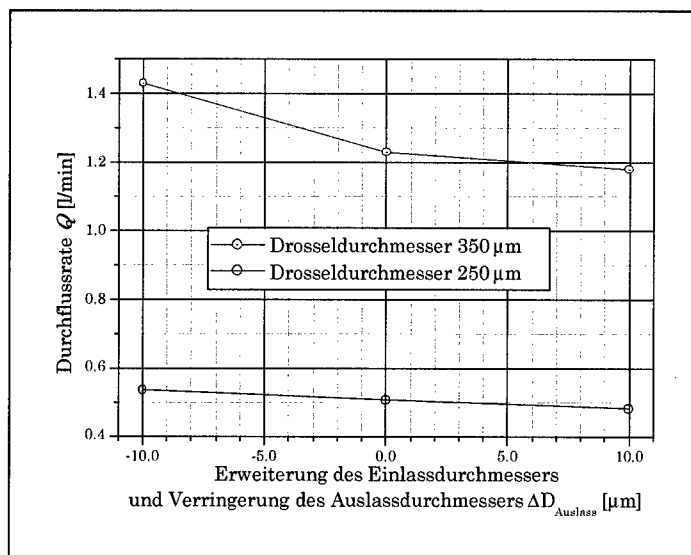
Abbildung 4.8: Durchfluss in Abhängigkeit von der Konizität. Der Einlass- und der Auslassdurchmesser wurden gegenläufig um 5 \mu\text{m} variiert. Drossellänge L = 1\text{ mm} ; Verrundungsradien jeweils 5% der Drosseldurchmesser am Ein- und Auslass. Rohrdurchmesser D_1 = 1\text{ mm} ; Drossellänge L = 1\text{ mm} .
