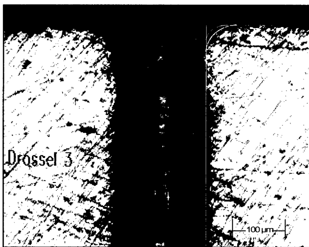
Abbildung 6.11: Profil einer Einlasskante mit einem Verrundungsradius von ca. 50 µm.
