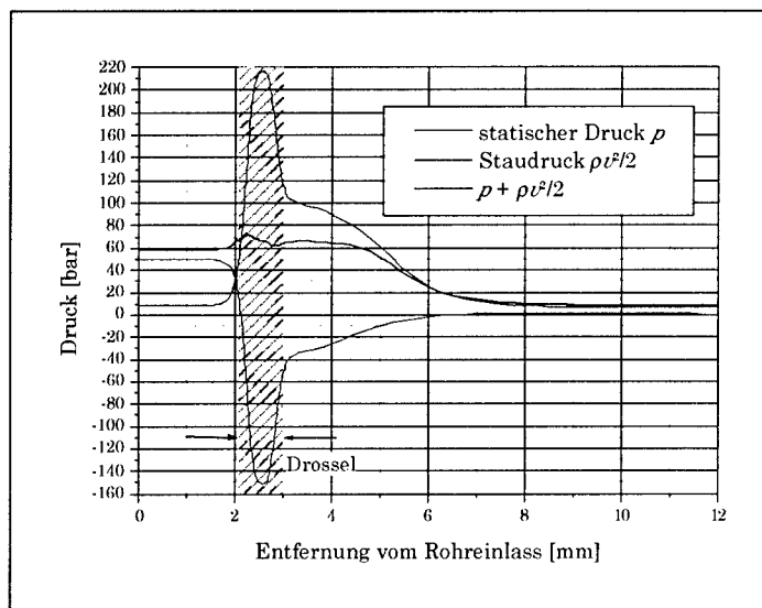
Abbildung 3.8: Entwicklung des statischen Drucks und des Staudrucks beim Durchströmen der Drossel. Bei einem Vordruck von 50 bar resultierte am Einlass auf Grund der Geschwindigkeit ein Staudruck von ca. 10 bar. Nach Bernoulli sollte die Summe der beiden Druckwerte konstant bleiben. Ab etwa 1 mm hinter der Drossel nimmt dieser Wert ab, was auf turbulente Verluste hindeutet.
