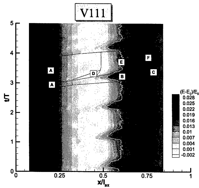
Abb. 5.17: Phasengemittelte Weg-Zeit-Diagramme der Quasi-Wandschubspannungen für die beiden Verdichtergitter bei Ma_1=0.15 , Re_1=200000 , t_{BAR}=80 mm, u_{BAR}=20 m/s
