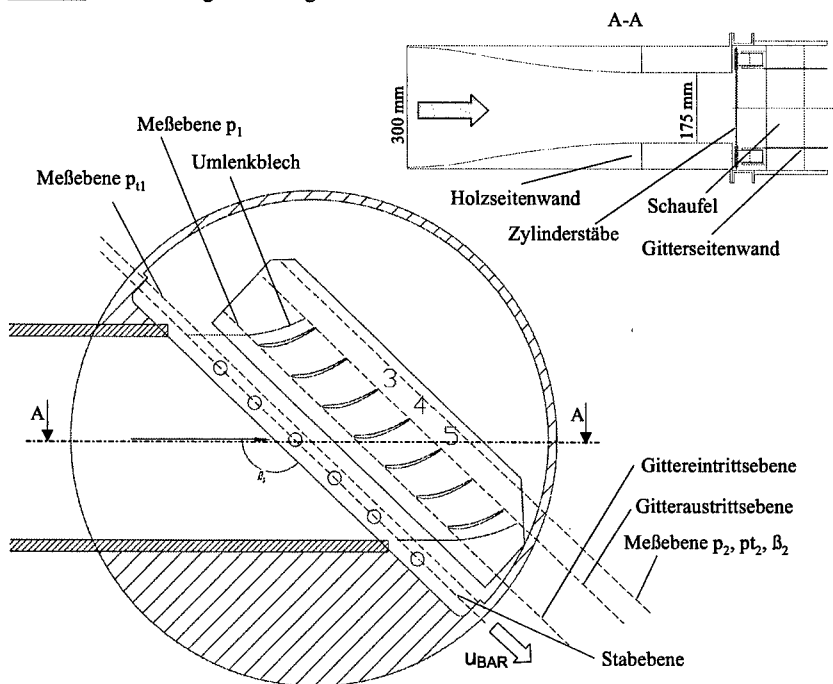
Abb. 3.2: Einbauskeizze des Verdichtergitters V111 in die Meßstrecke des HGK
