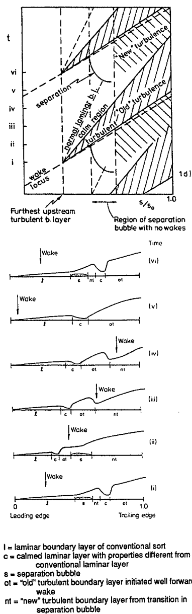
Abb. 2.10: Schematischer Verlauf der Grenzschichtdicke in verschiedenen Zeitschnitten während einer Dellendurchlaufperiode auf der Saugseite einer Verdichterschaufel (Cumpsty et al. 1995)
