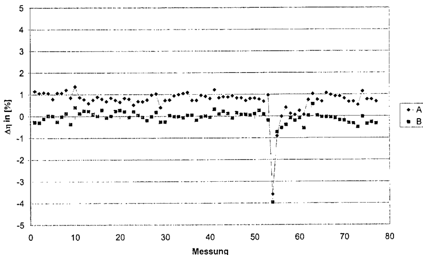
Abb. 4.10: Wirkungsgradveränderung.
