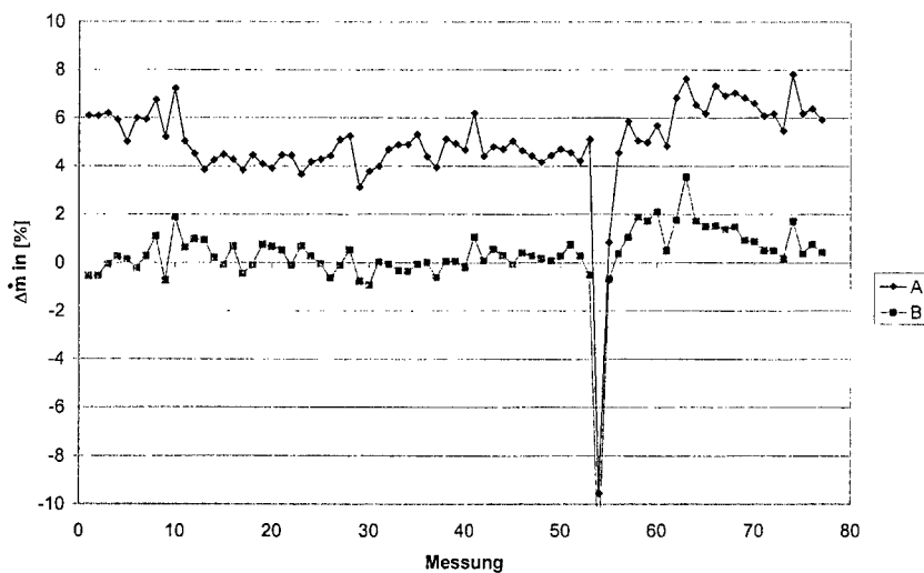
Abb. 4.11: Normierter Leckagemassenstrom.
