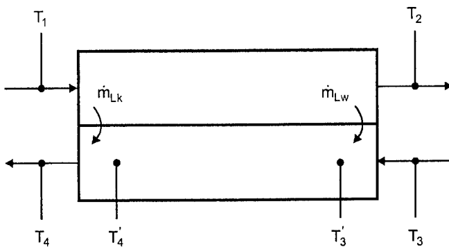
Abb. 2.3: Temperaturkorrektur.
