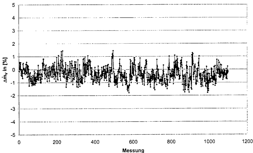
Abb. 4.7: Massendurchsatz des Axialverdichters (1 Matrix, belastungsabhängiger Referenzpunkt).
