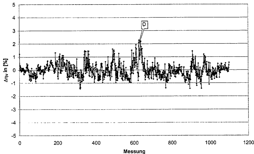
Abb. 4.6: Wirkungsgrad des Axialverdichters (1 Matrix, belastungsabhängiger Referenzpunkt).
