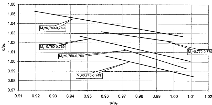
Abb. 4.3: normiertes \phi - \psi -Kennfeld des Axialverdichters (Berndt, 2000).
