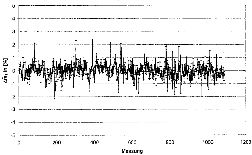
Abb. 4.20: Turbinendurchsatz.
