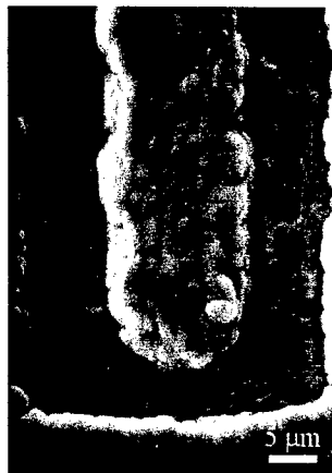
Abbildung 2.9: REM-Aufnahme einer Interdigitalelektrode mit Ga 2 O 3 besputtert
