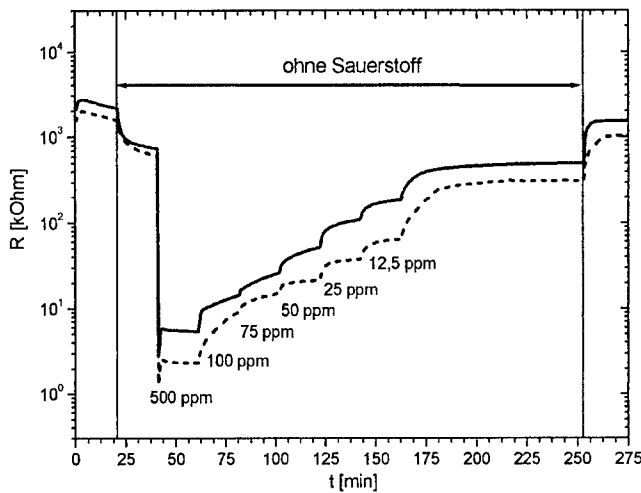
Abb. 5.3: Widerstandsverlauf von zwei Standard- H_2 -Sensoren auf verschiedene Konzentrationen von Wasserstoff in feuchtem (20% r.F.), sauerstofflosem Gasgemisch bei einer Betriebstemperatur von 700^\circ\text{C}
