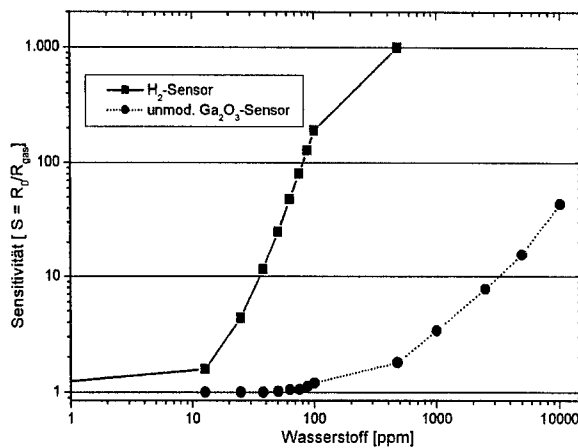
Abb. 5.1: Vergleich der Sensitivität auf Wasserstoff zwischen einem Standard-H 2 -Sensor und einem unmodifizierten Ga 2 O 3 -Sensor bei einer Betriebstemperatur von 650°C in feuchter (20% r.F.), synthetischer Luft
