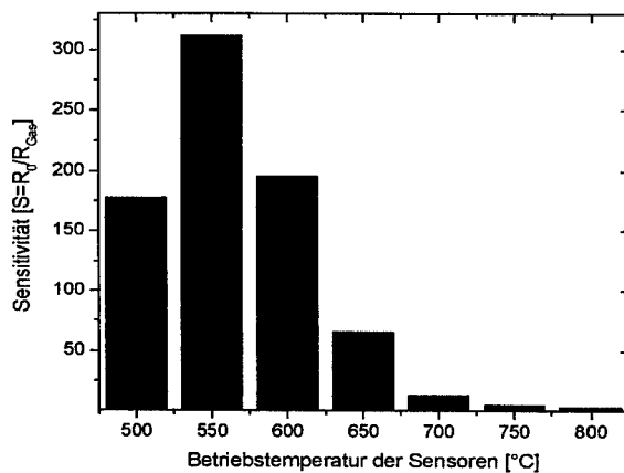
Abb. 3.15: Wasserstoffsensitivität auf eine Konzentration von 100 ppm H 2 in Abhängigkeit der Betriebstemperatur von H 2 -Sensoren mit einer bei 1050°C getemperten Ga 2 O 3 -Schicht in feuchter, synthetischer Luft
