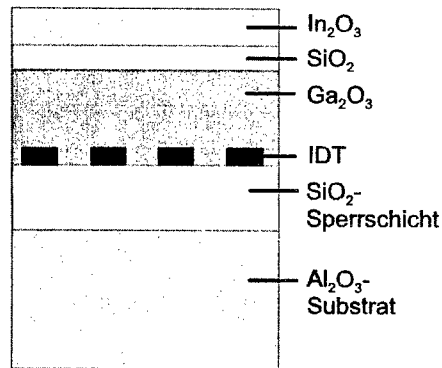
Abb. 4.9: Prinzipdarstellung des Schichtsystems der \text{In}_2\text{O}_3 -Filterschichtsensoren
