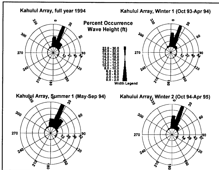
Figure 17. Wave height roses, Kahului array
