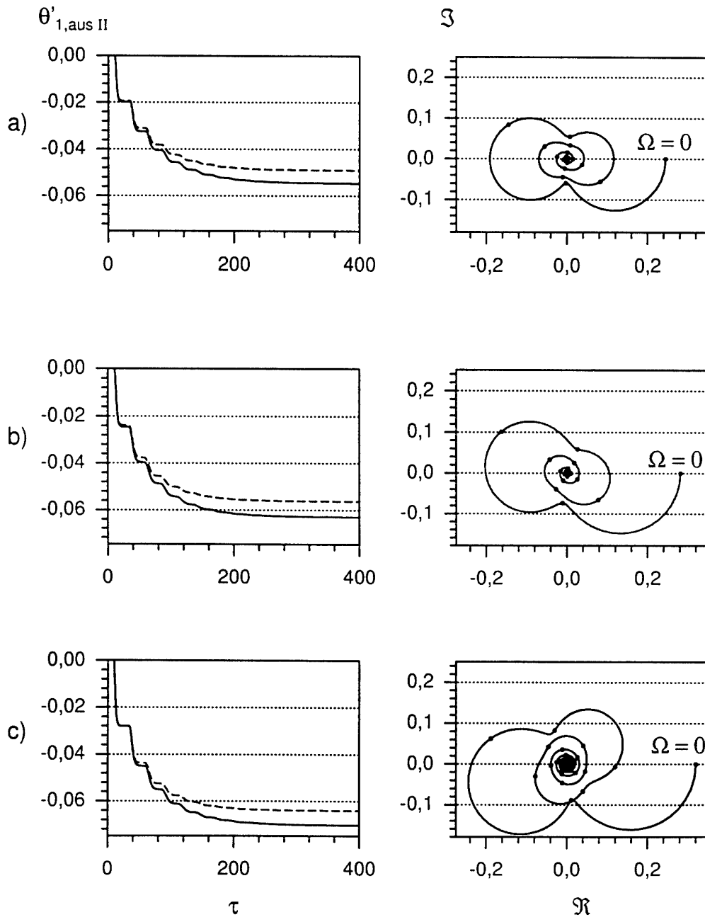
Abb. 7.11. Systemantwort auf eine Schwankung des Massenstroms des Hauptstroms I. a) Kreuzstrom mit quervermischt Umlaufstrom, b) Kreuzstrom mit quervermischten Hauptströmen, c) Gegenstrom. Links Sprungantworten (die Lösung der exakten Energiegleichungen ist durchgezogen, die der linearisierten Energiegleichungen gestrichelt), rechts Frequenzgänge. Der Abstand zwischen den markierten dimensionslosen Kreisfrequenzen beträgt \Delta\Omega = 2\pi/50 .
