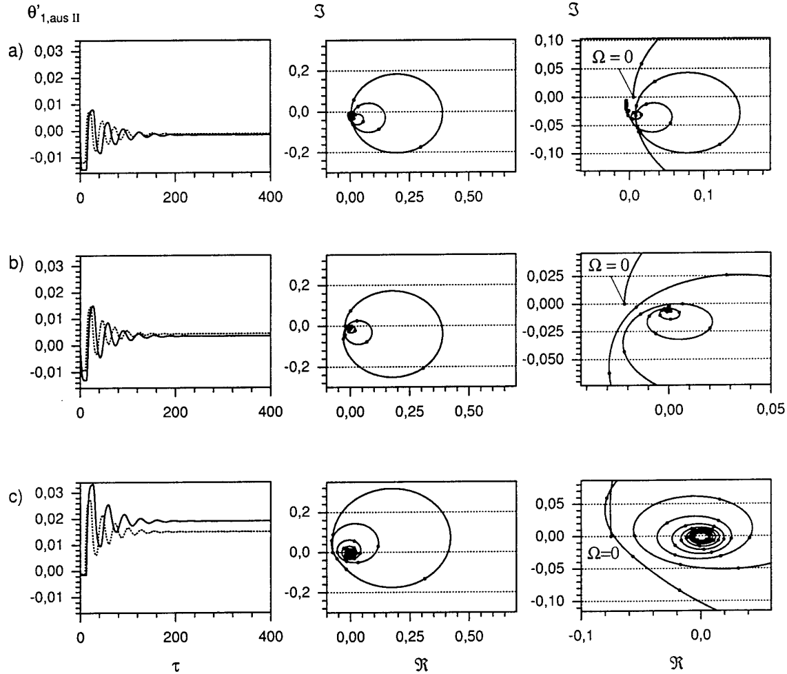
Abb. 7.13. Systemantwort auf eine Schwankung des Massenstroms des Umlaufstroms. a) Kreuzstrom mit quervermishtem Umlaufstrom, b) Kreuzstrom mit quervermischten Hauptströmen, c) Gegenstrom. Links Sprungantworten (die Lösung der exakten Energiegleichungen ist durchgezogen, die der linearisierten Energiegleichungen gestrichelt), Mitte und rechts Frequenzgänge. Der Abstand zwischen den markierten dimensionslosen Kreisfrequenzen beträgt \Delta\Omega = 2\pi/50 .
