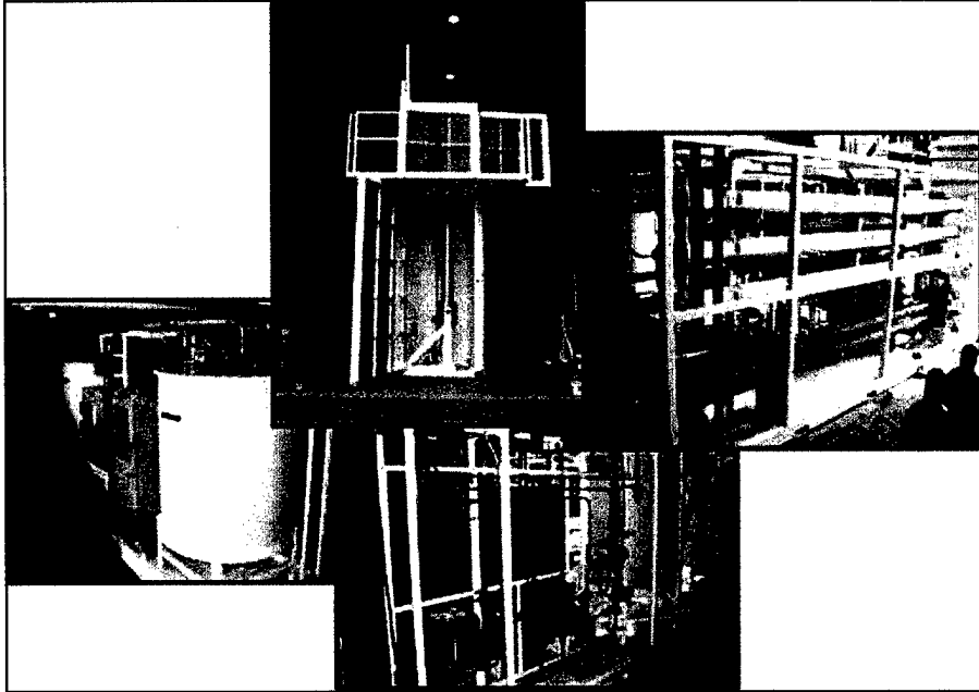
Fig. 2-7. ROK SCWO system (McAlester, OK)
