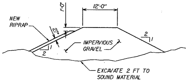
NEW LEVEE
