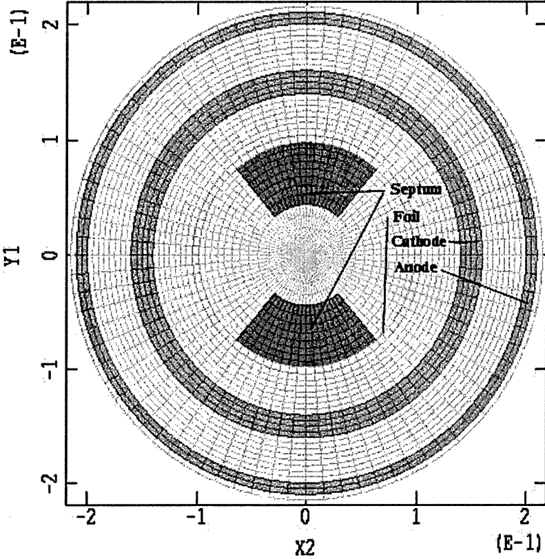
Figure 16 Enlarged smooth edge septum.
