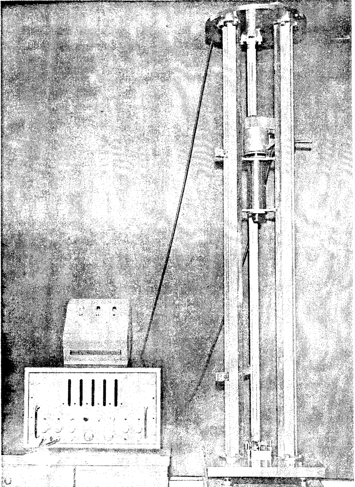
Fig. 1 Impact Tester
