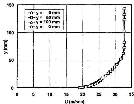
a) Mean longitudinal flow
