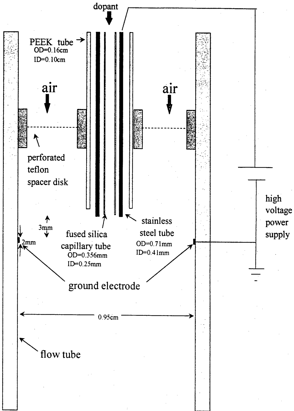
Fig. 1. Electrospray apparatus.
