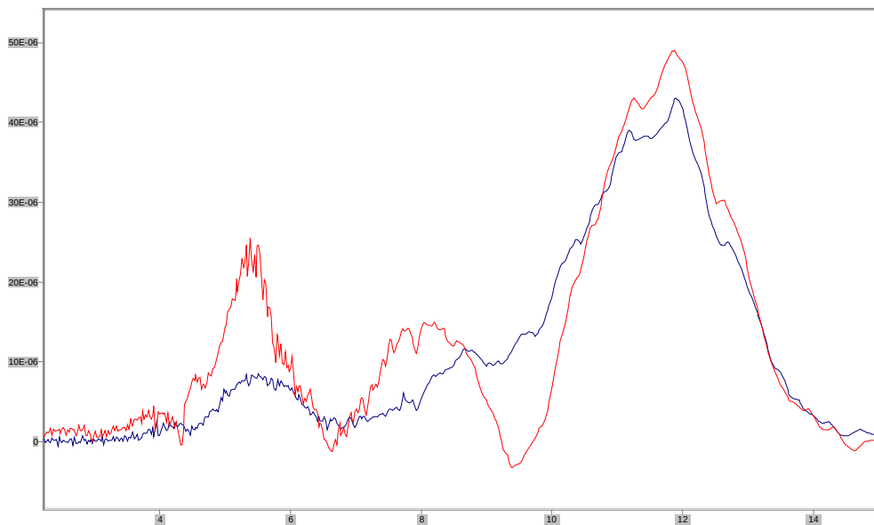
Graph III-1: RS-40 Open Burn IR Spectra
