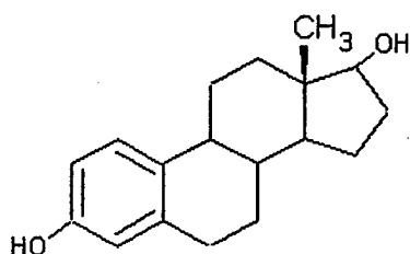
1,3,5(10)-estratrien-3, 17 beta-diol
