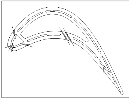
Figure n°3 : Snecma Moteurs 2 nd advanced wall cooling circuit
