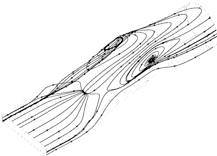
Abb. 7.14: Wandnahe Stromlinien, Rechnung FINE/Turbo, k - \epsilon -Modell, Modifikation YANG
