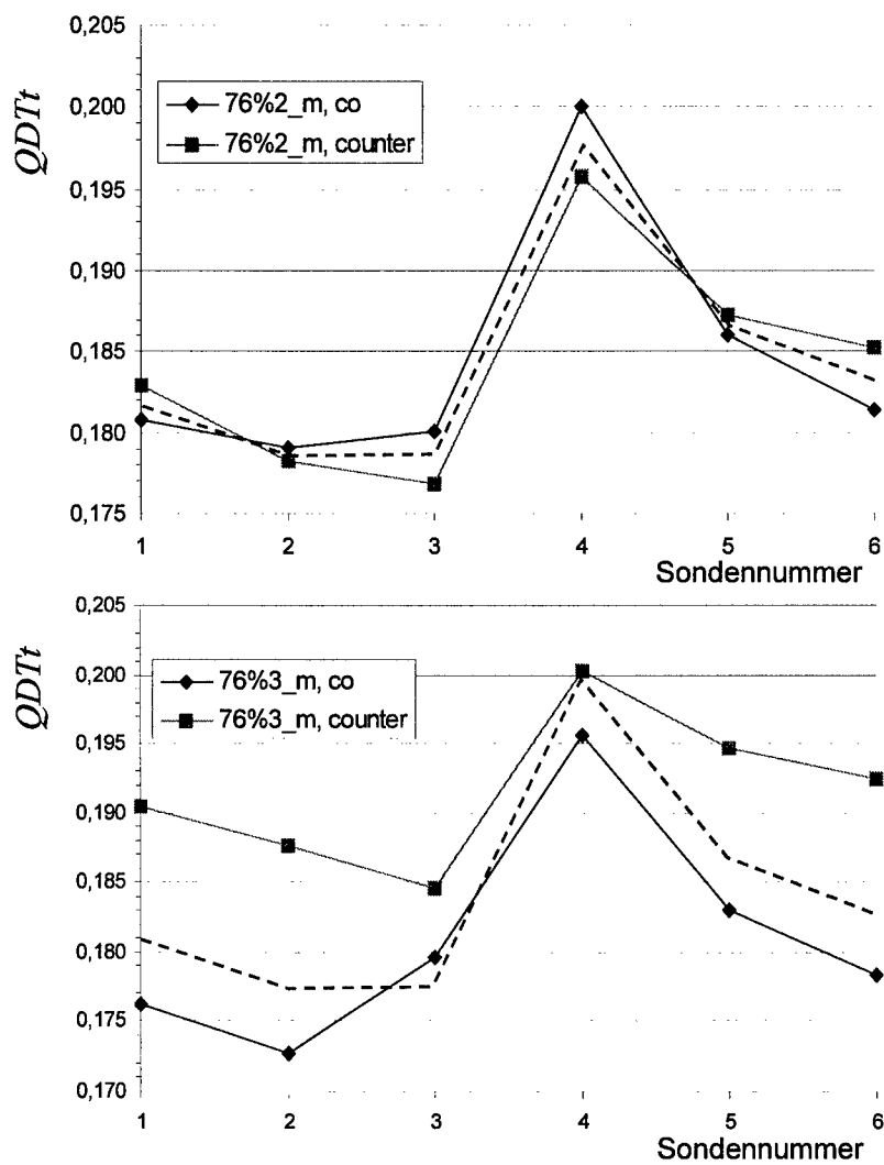
Abb. 6.12: Verlauf der radial aufgelösten Totaltemperaturen T_{t21} : n_{red,NDV}=76\% ; Sonde 1: Gehäuse, Sonde 6: Nabe
