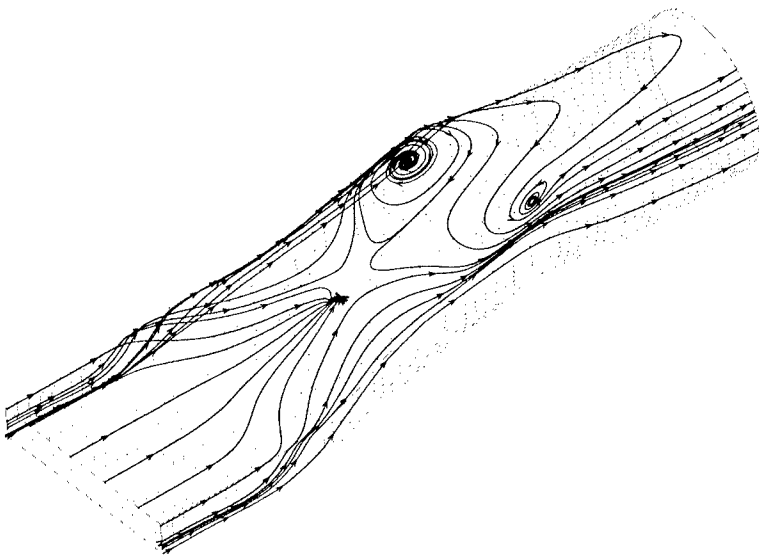
Abb. 7.13: Wandnahe Stromlinien, Rechnung FINE/Turbo, k - \epsilon -Modell, Modifikation CHIEN
