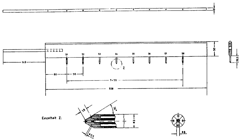
Abb. 4.12: Schemazeichnung des Drallmeßrechens und einer Einzelsonde
