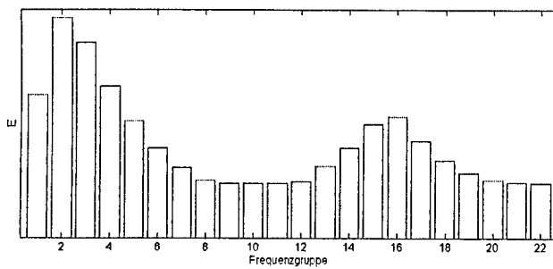
Abbildung 5.16.: Erregungsverteilung eines Signalsegmentes über die 22 gehörrechtlichen Tonheitskanäle. Durch die beschriebene Faltungsoperation jedes Frequenzgruppenspektrums gem. Abbildung 5.12 mit der Schablone gem. Abbildung 5.14 bzw. 5.15 entsteht pro Kanal ein diskreter Wert, der mit der psychoakustischen Erregung des menschlichen Gehörs korrespondiert.
