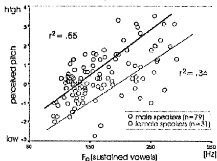
Abbildung 4.39.: Zusammenhang zwischen Messungen des mittleren Pitch an isolierten Vokalen (Abszisse) und perzeptiven Hörer-Ratings anhand des natürlichen Redeflusses (Ordinate), getrennt nach weiblichen und männlichen Patienten.
