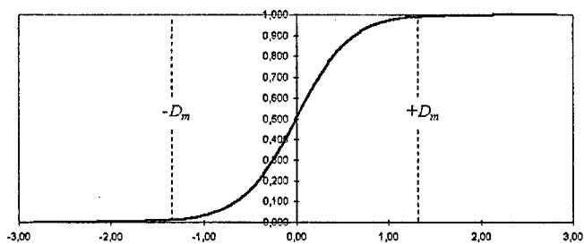
Abbildung 7.27.: Abschnittsweise definierte Rückschlußwahrscheinlichkeit zur Klasse der Frikative in Abhängigkeit des Diskriminanzscores D
