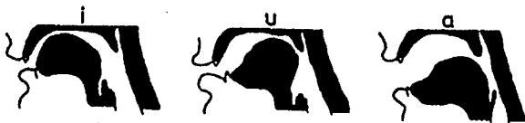
Abbildung 1.5.: Stellung des Artikulationstraktes und der Zunge bei den Vokalen /i/ (links), /u/ (mitte) und /a/ (rechts). Der Vokal /y/ (nicht dargestellt) unterscheidet sich von /i/ nur durch eine Vorstülpung der Lippen ([Fel84]).
