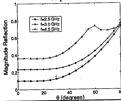
H-plane scan
